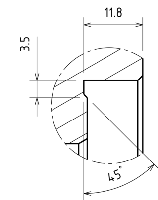
Detail B Scale: 4:3
