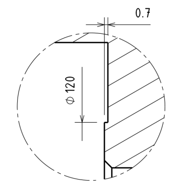
Detail C Scale: 4:3
