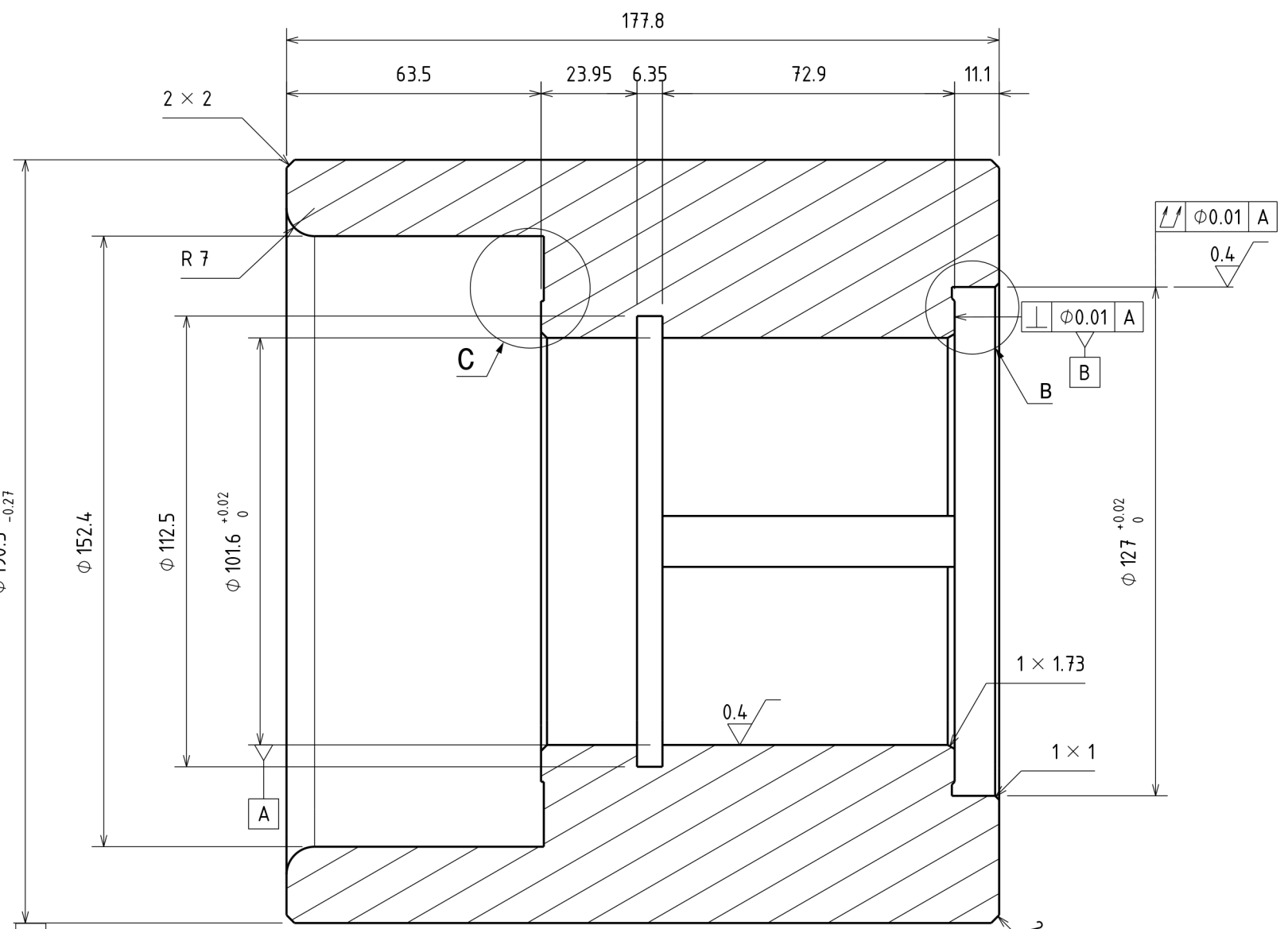
Section view A-A Scale: 2:3
