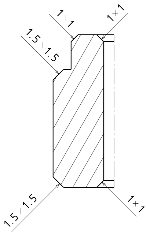
Detail B Scale: 3:1
